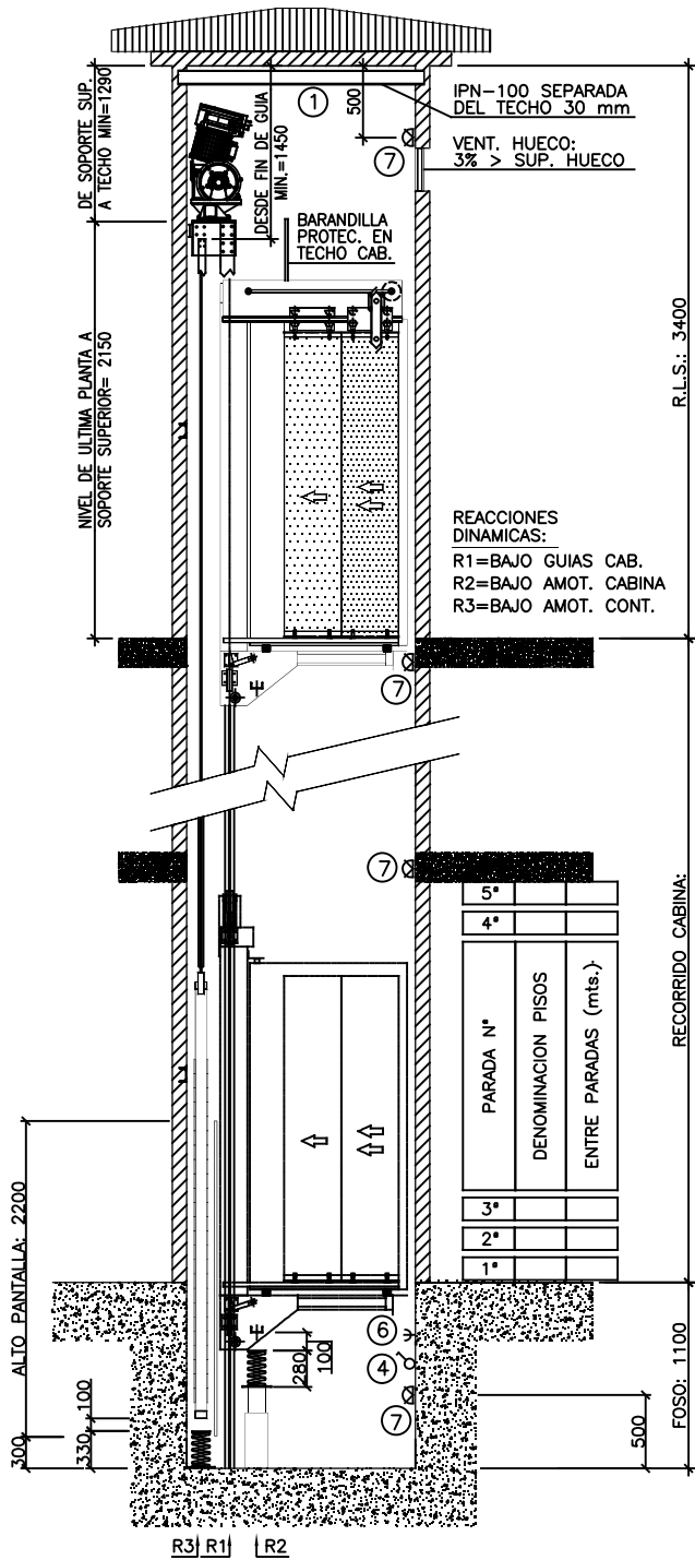
ALZADO
