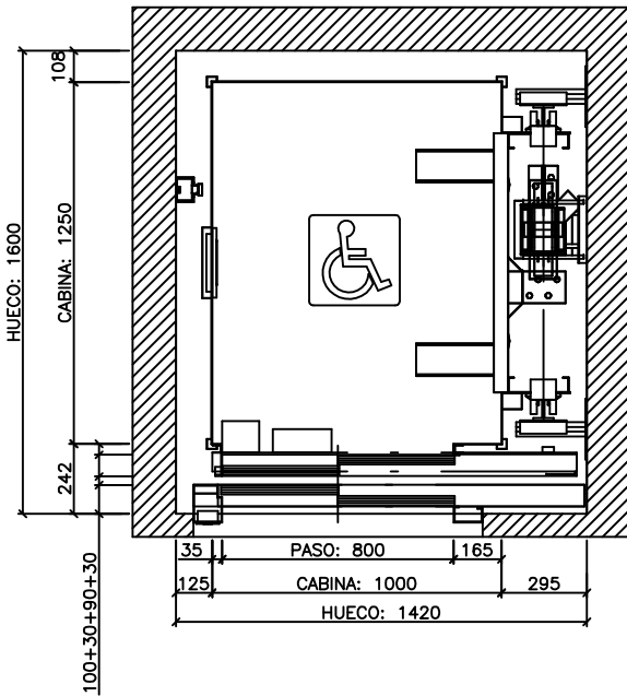
PLANTA DE PISOS
